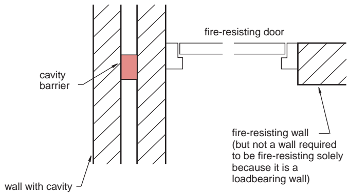
(d) Plan
